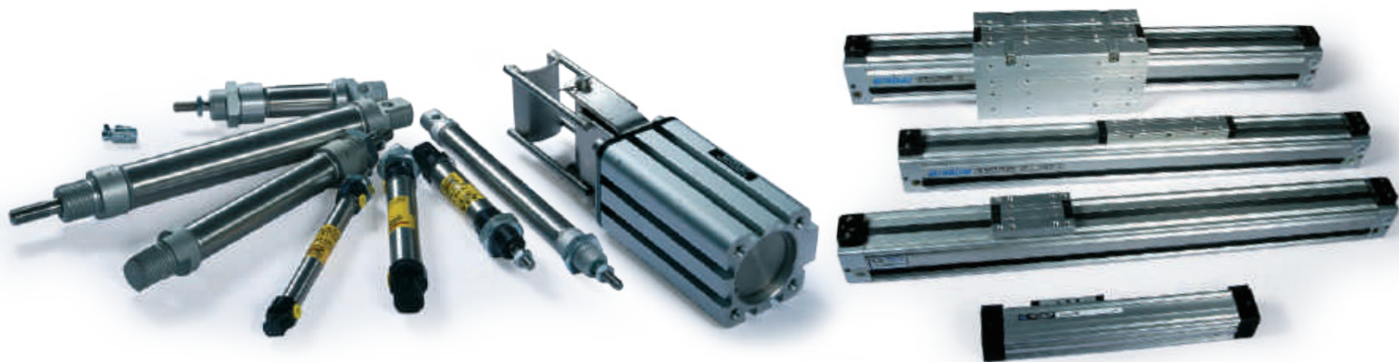
Cilindri: okrogli, pnevmatski, klasični, kompaktni, rotacijski, z nevtljivo batnico.
